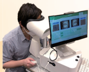
視野検査
